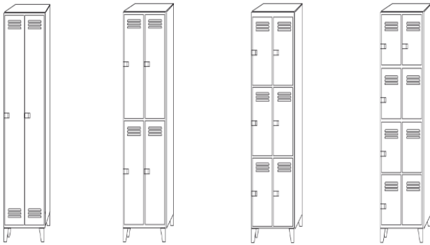
Modelo: LK-21 2 Cuerpos 2 Puertas Modelo: LK-24 2 Cuerpos 4 Puertas Modelo: LK-26 2 Cuerpos 6 Puertas Modelo: LK-28 2 Cuerpos 8 Puertas
